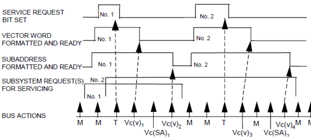
ASYNCHRONOUS MESSAGE (SUBADDRESS) REQUEST
