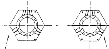
Inch Conelock Nuts
