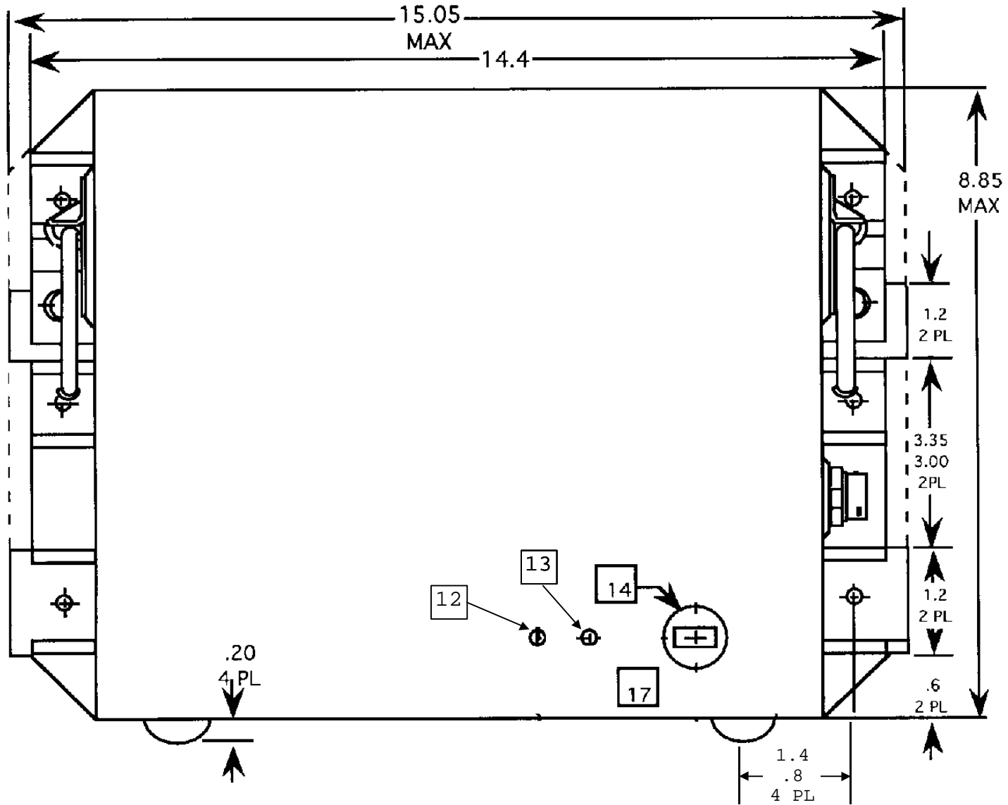
FIGURE F-2. DRUH front.
